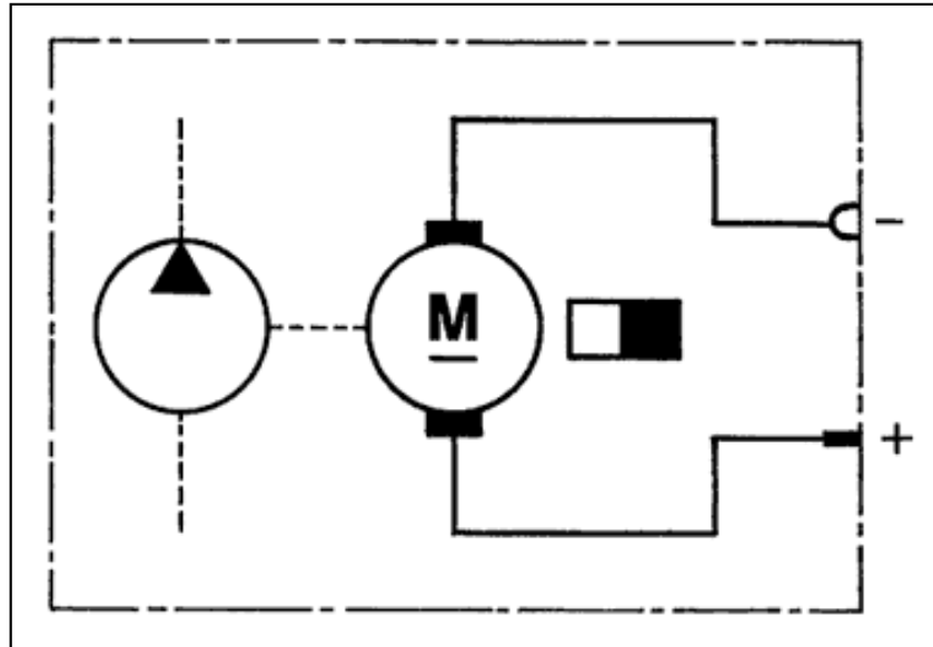
Abb.: Anschlussbild Bestell-Nr. 0 392 040 008
